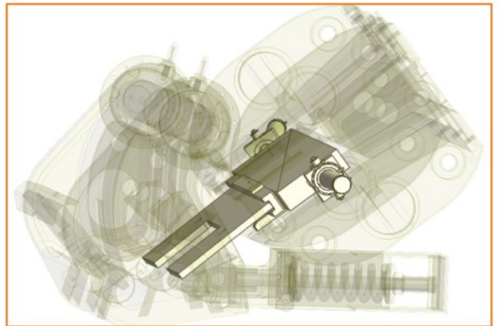
破碎間隙自動調整機構 Automatic discharge set adjustment
